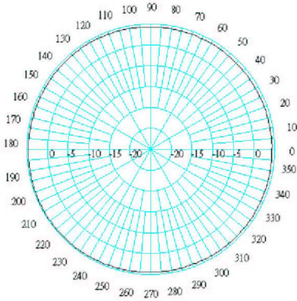
H-PLANE 2.45GHZ=4.876dbi
